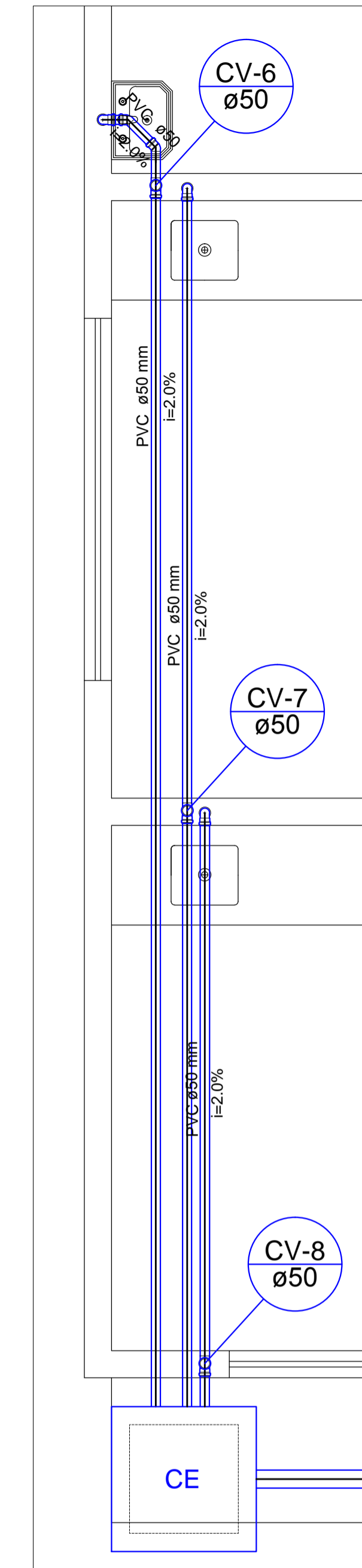
5 DETALHE S3 ESCALA 1:25
