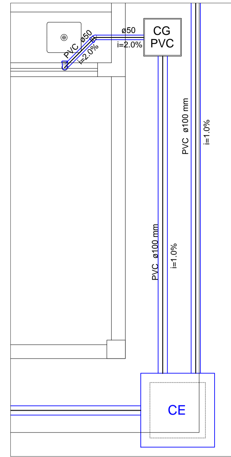
2 DETALHE S5 ESCALA 1:25
