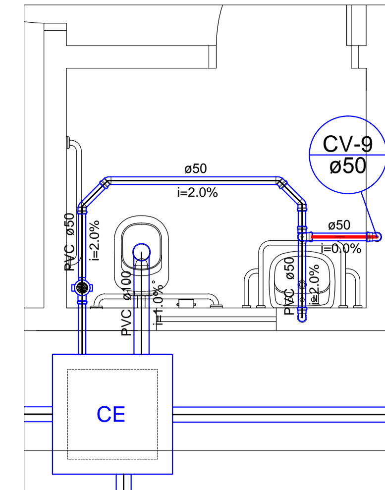
4 DETALHE S4 ESCALA 1:25
