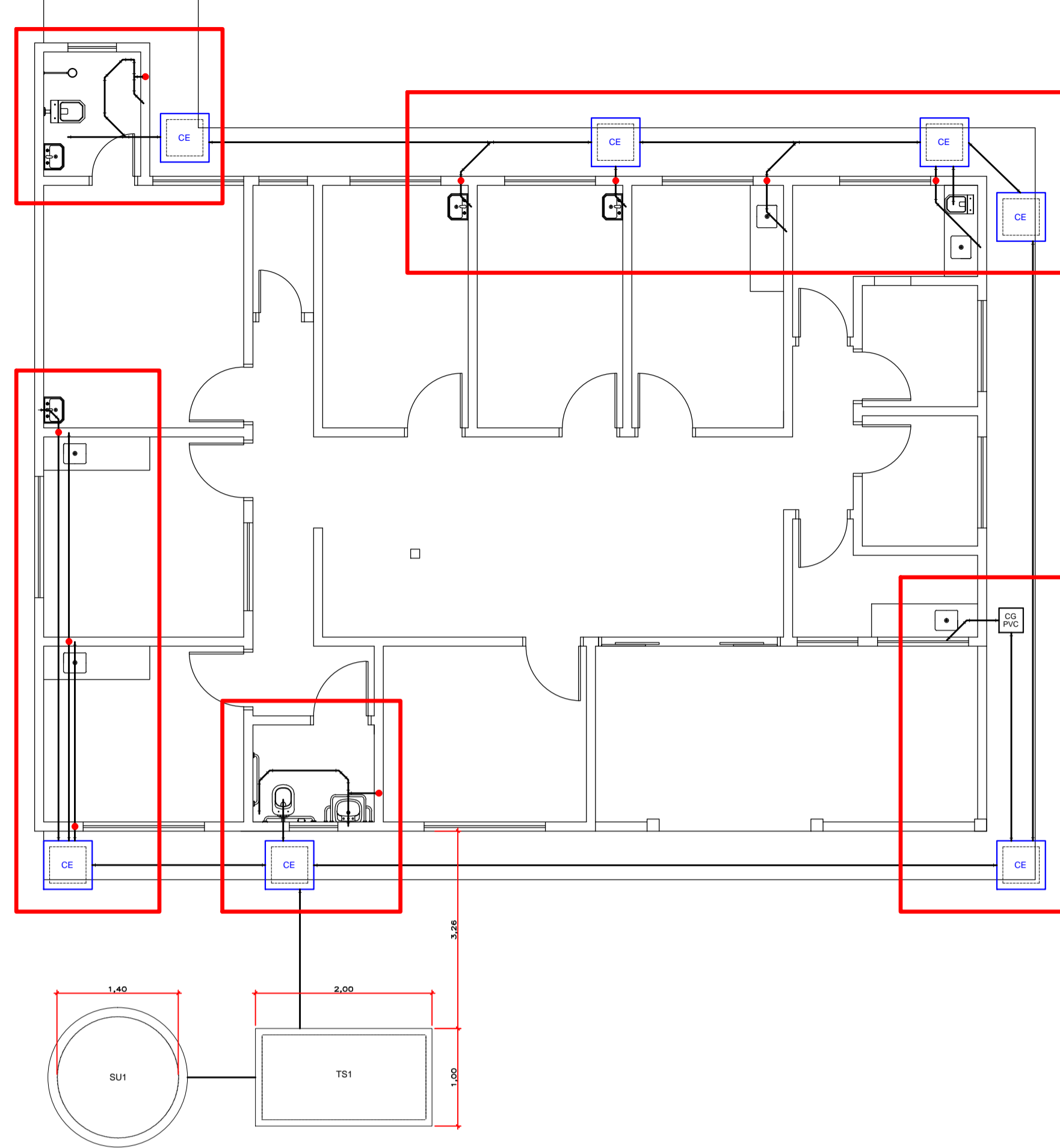
1 PLANTA BAIXA PROJETO DE ESGOTO SANITÁRIO ESCALA 1:75
