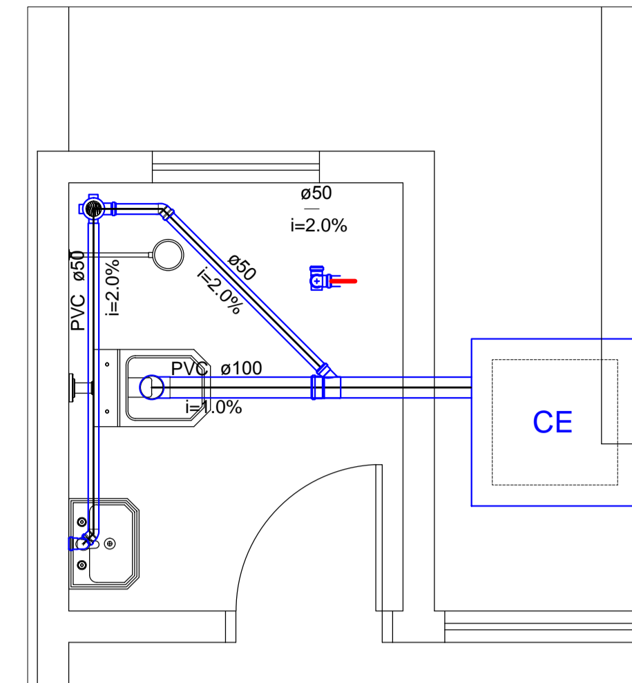
3 DETALHE S1 ESCALA 1:25
