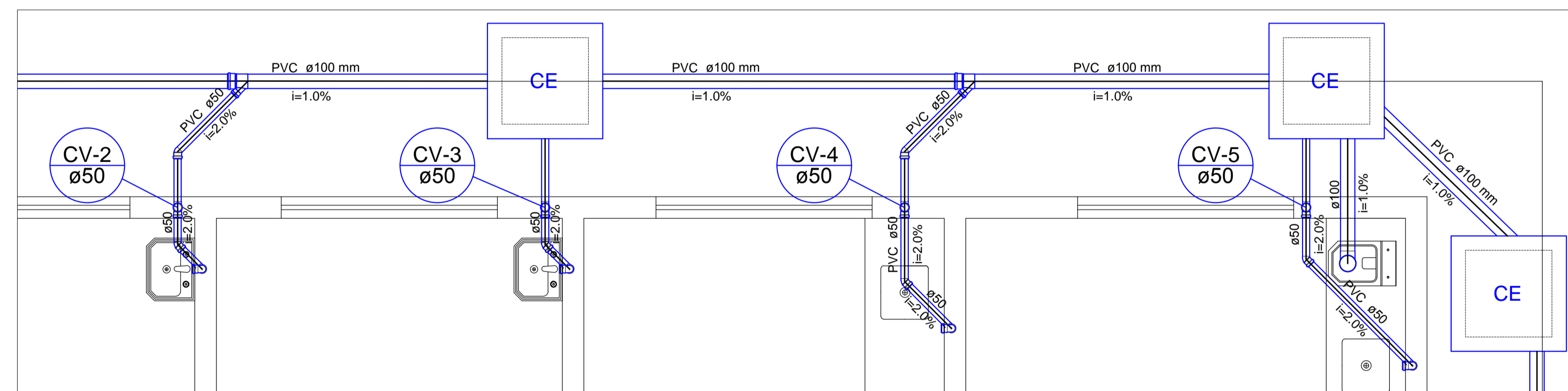
6 DETALHE S2 ESCALA 1:25
