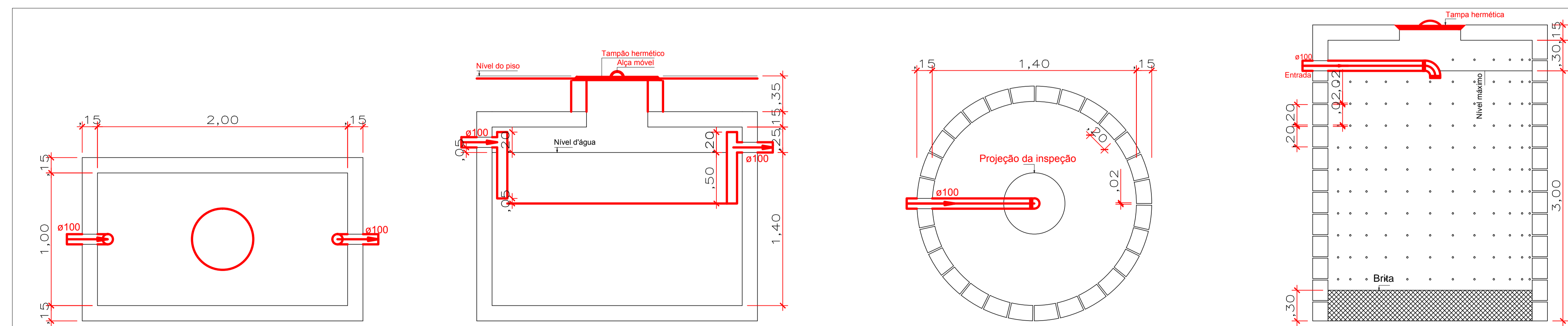
7 DETALHE UNIDADES DE TRATAMENTO ESCALA 1:25
